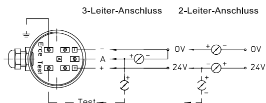
Bauform Feldgehäuse
