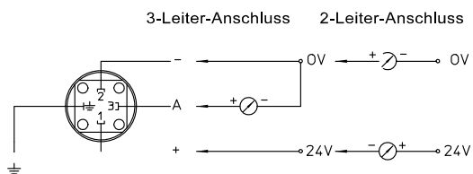
Bauform Standardgehäuse
