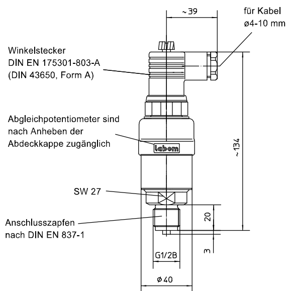
Bauform Standardgehäuse
