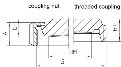
Sanitary pipe connection per DIN 11851 for pipes per EN 10357
